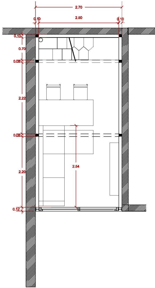
PLANTA 1
