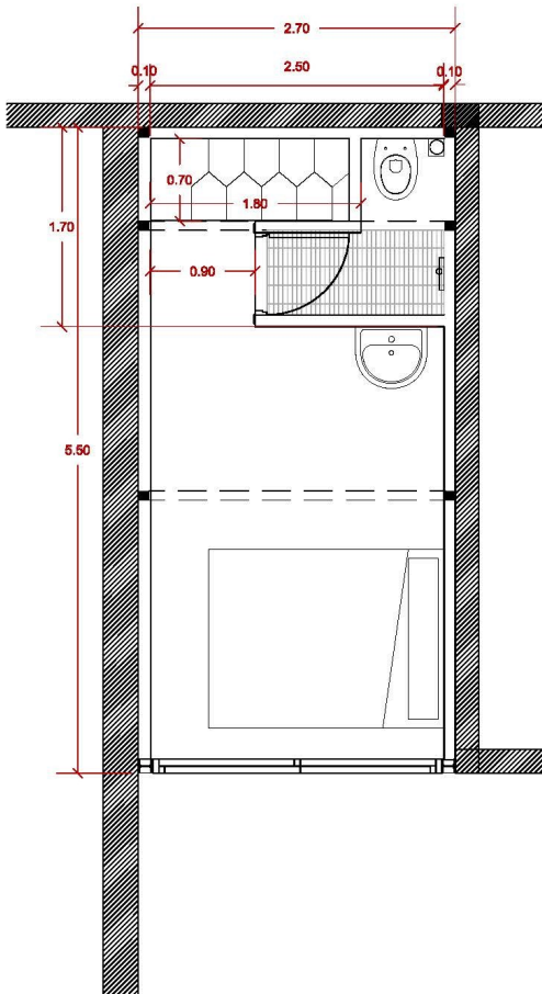
PLANTA 2
