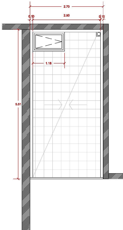
PLANTA CUBIERTA
