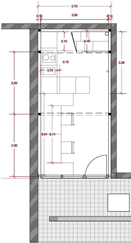
PLANTA 0
