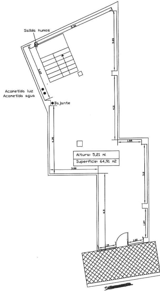
PLANTA BAJA
