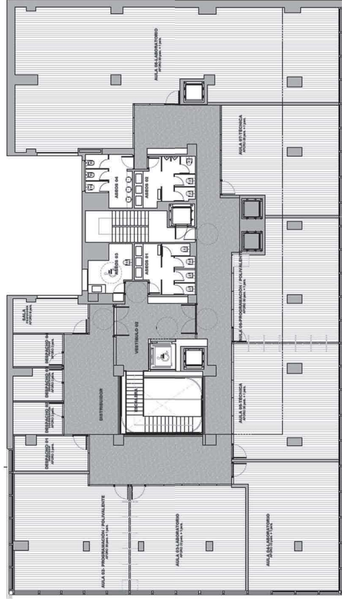
DISTRIBUCIÓN INTERIOR PLANTA PRIMERA
