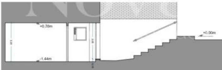
SECCIÓN B-B
