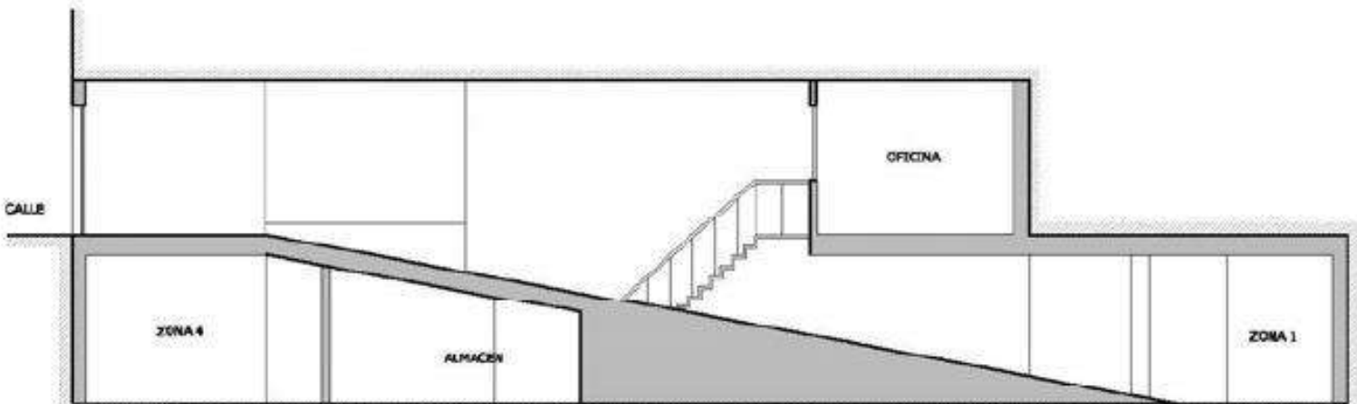
Sección Rampa
