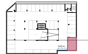
NIVEL GARAJE 03 PLANTA N -16.50 ESCALA 1:500
