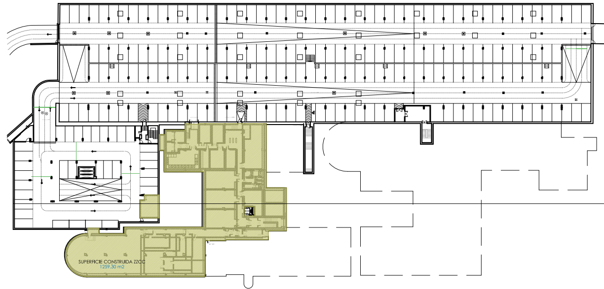
NIVEL -02/GARAJE 01 PLANTA N -8.00 ESCALA 1:500
