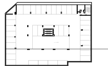
NIVEL GARAJE 02 PLANTA N -13.40 ESCALA 1:500
