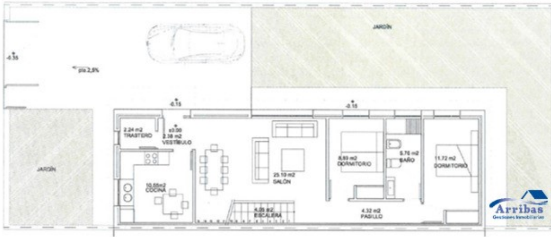
PLANTA BAJA ESC 1/100
