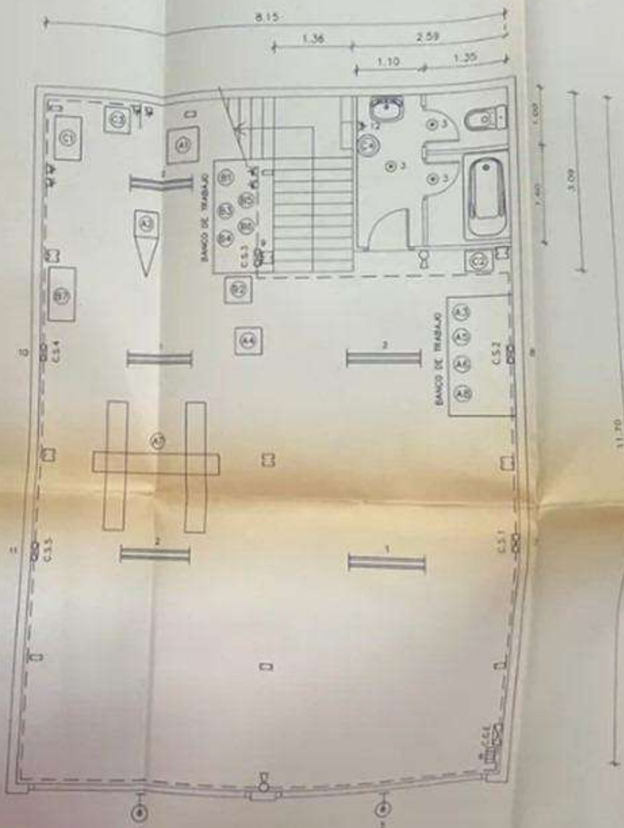
PLANTA BAJA
