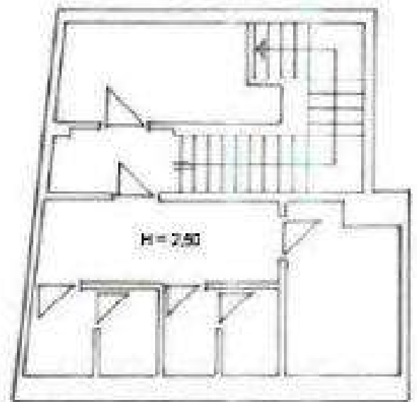
PLANTA SOTANO
