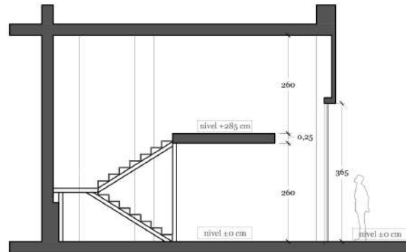
SECCIÓN TRANSVERSAL
