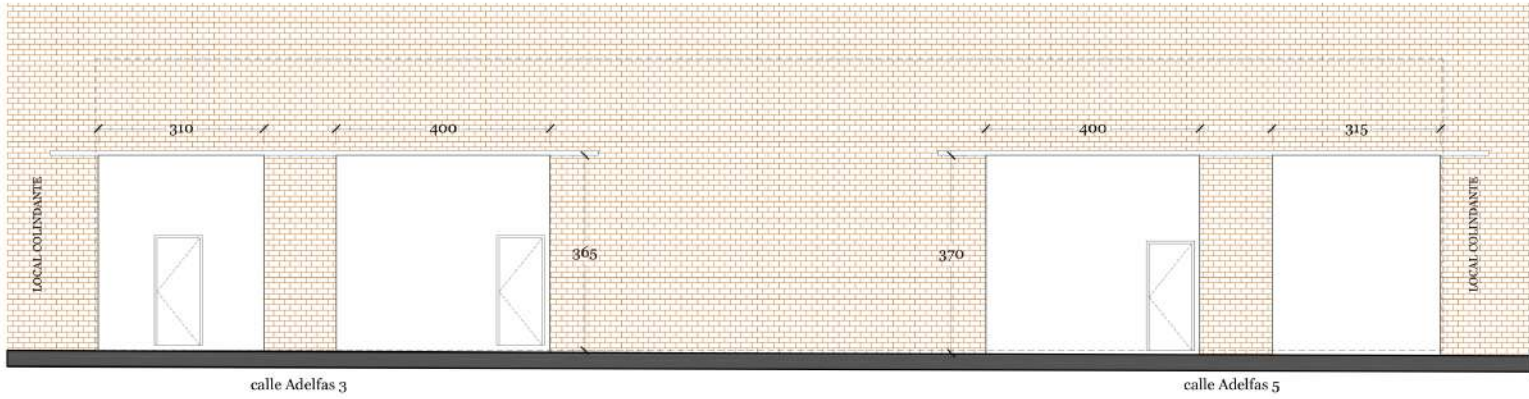
ALZADO
