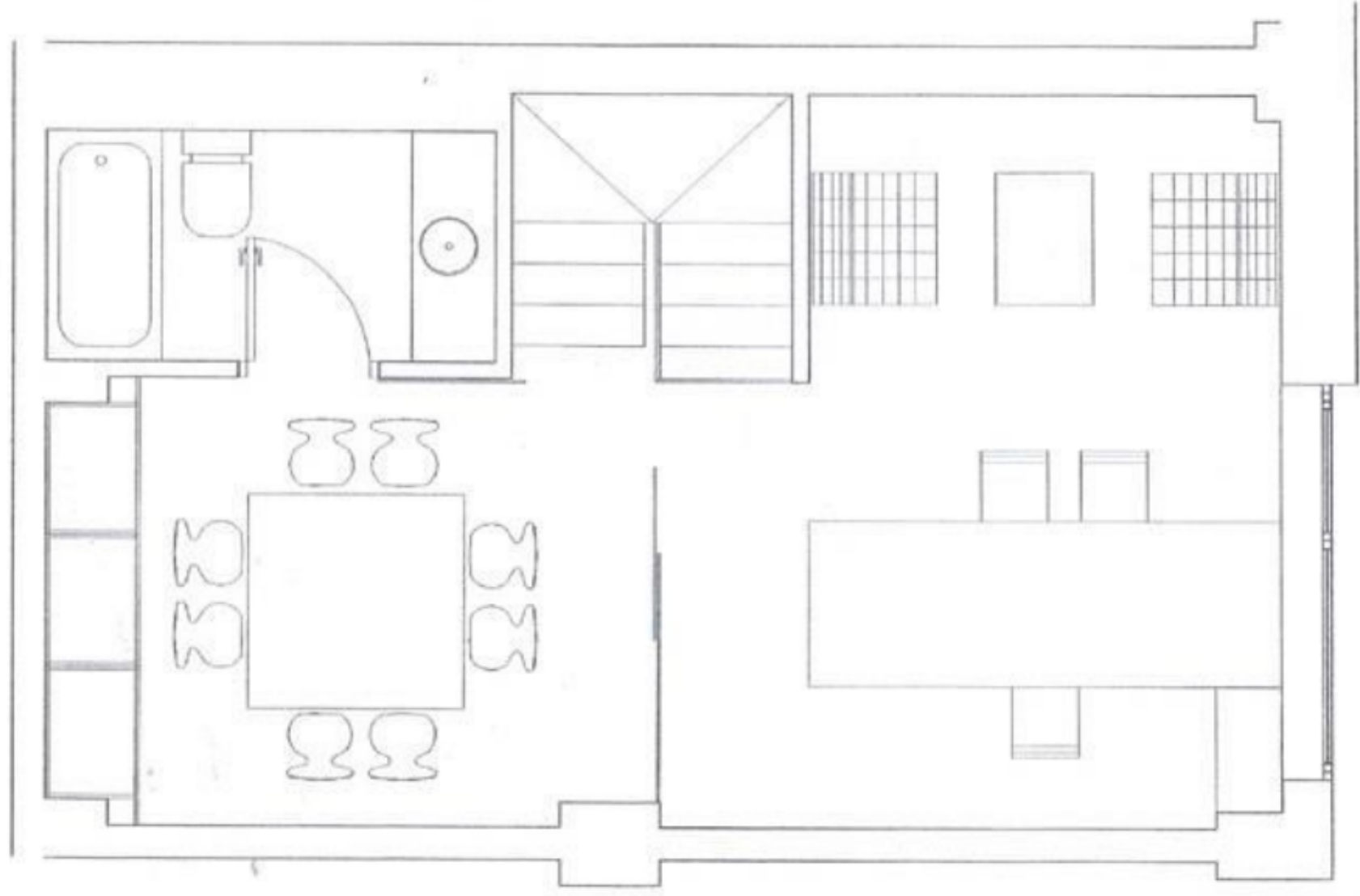
pianta alta proposta a:1/50
