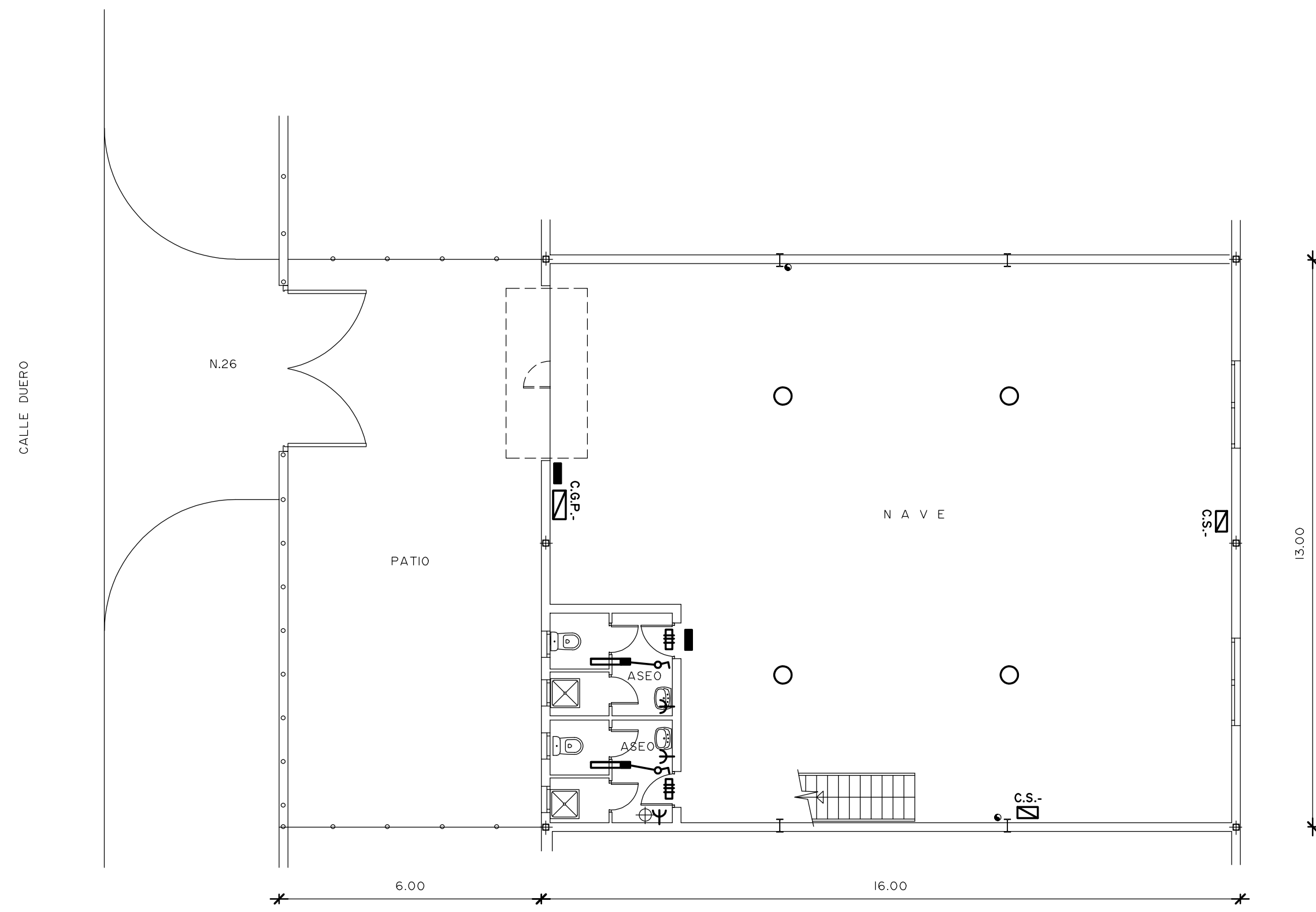
PLANTA BAJA
