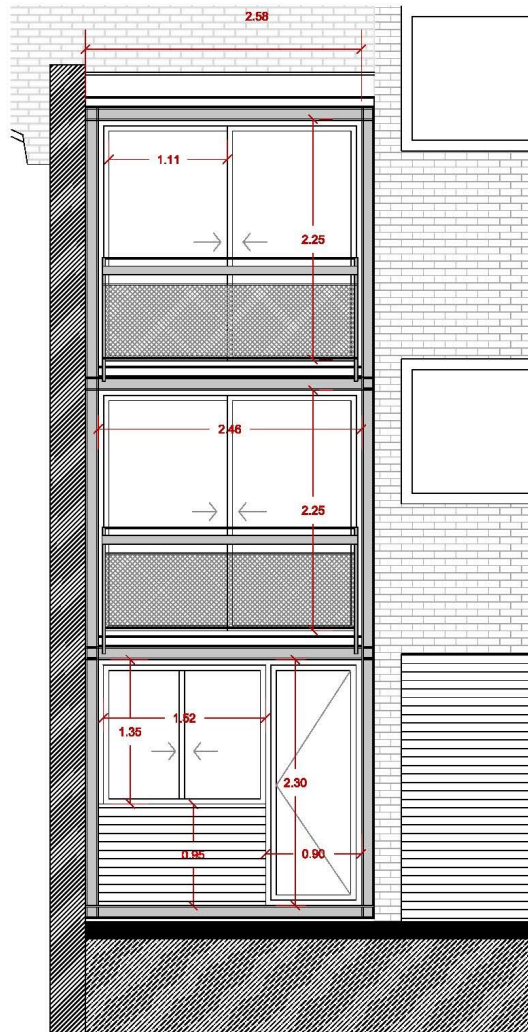
ALZADO
