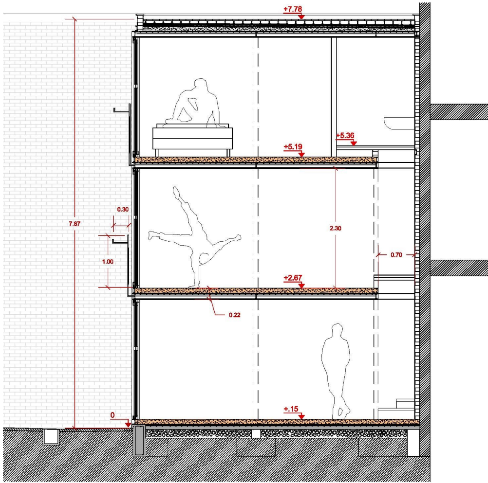
SECCIÓN LONGITUDINAL
