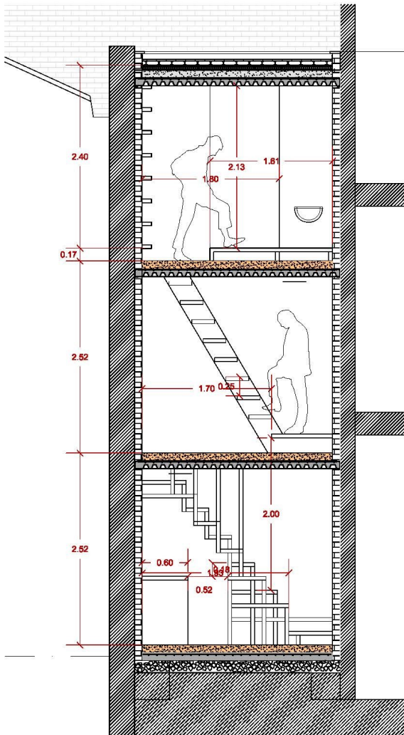
SECCIÓN TRANSVERSAL
