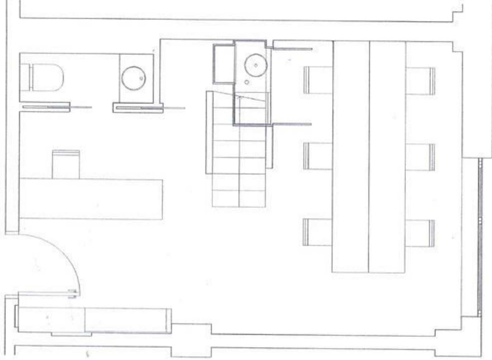
planta baja propuesta e: 1/50
