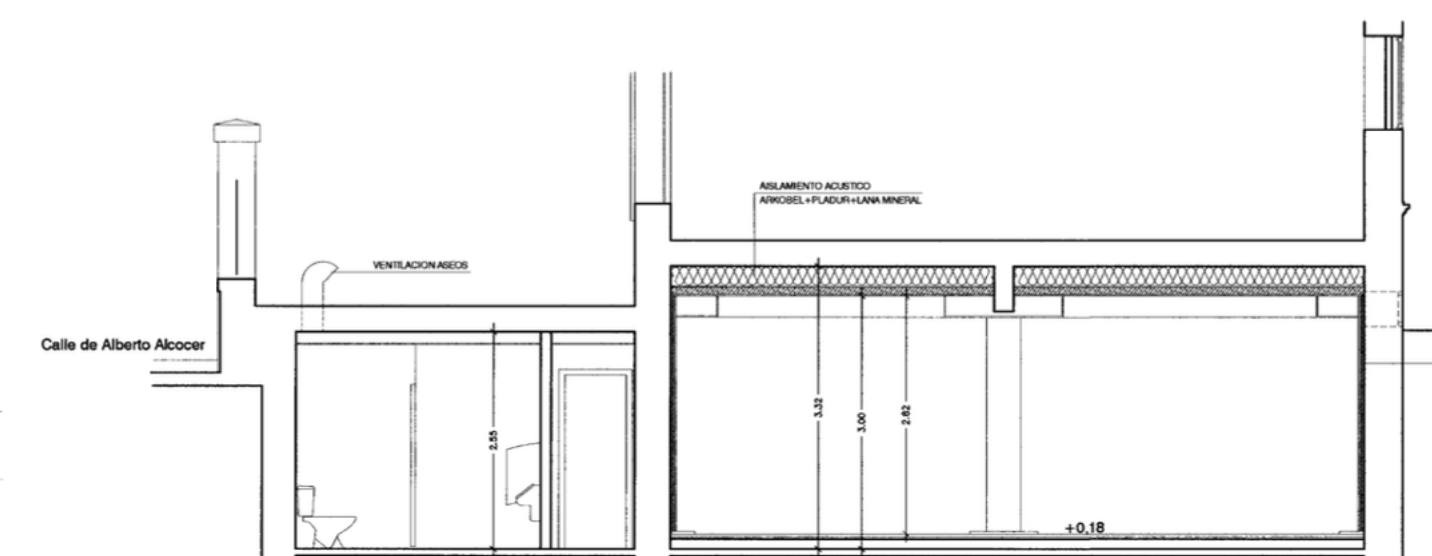
SECCION C-C
