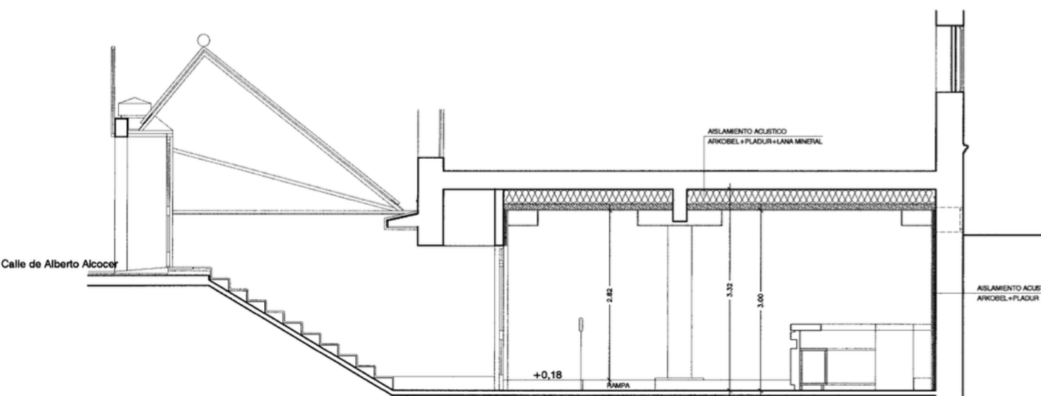
SECCION B-B
