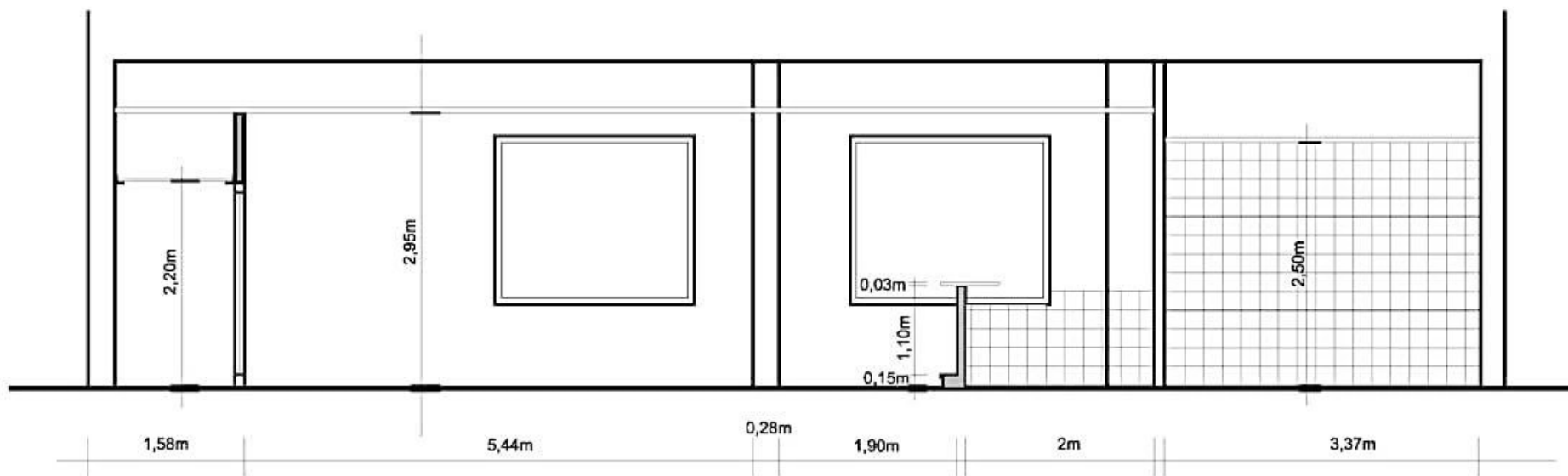
SECCIÓN. E:1/50
