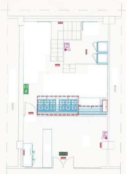
PLANTA BAJA
