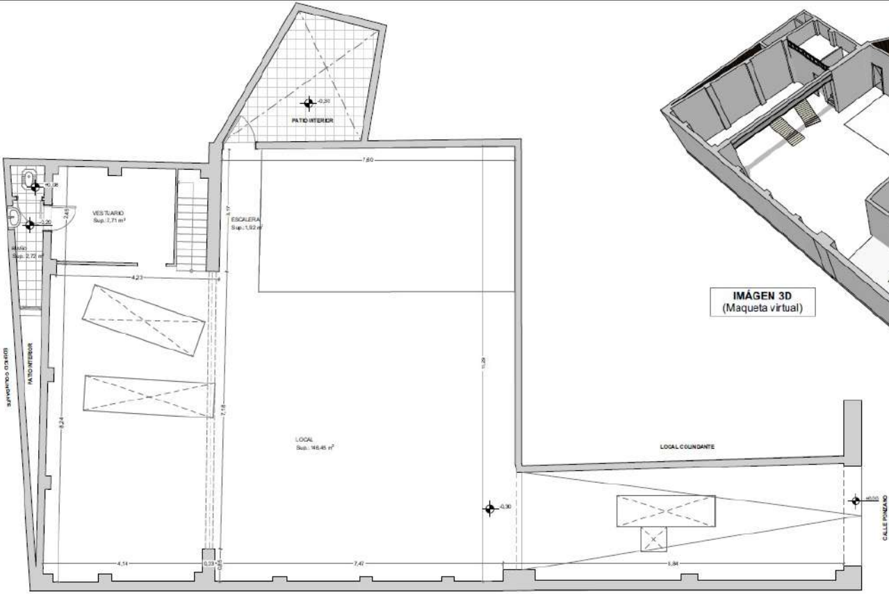
EDIFICIO COLINDANTE PLANTA ESTADO ACTUAL Escala 1:50
