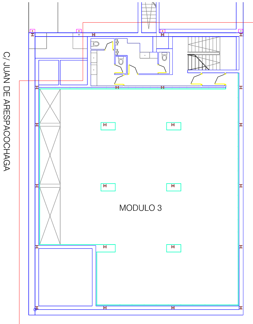
PLANTA SOTANO
