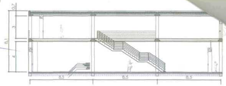
sección longitudinal 1/300
