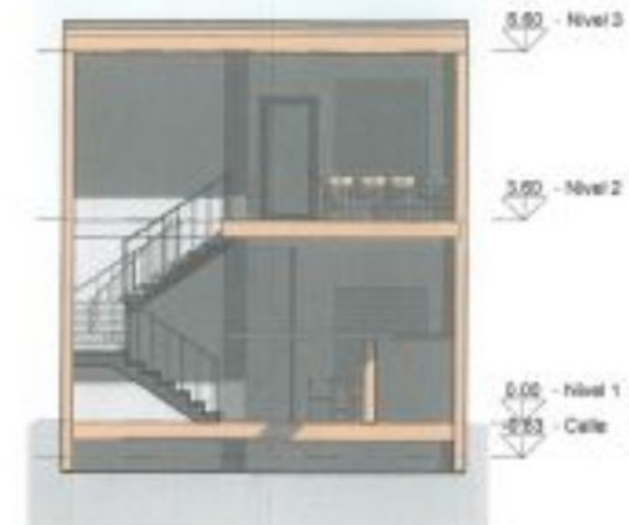
3 Sección 4 Alto: 1:100
