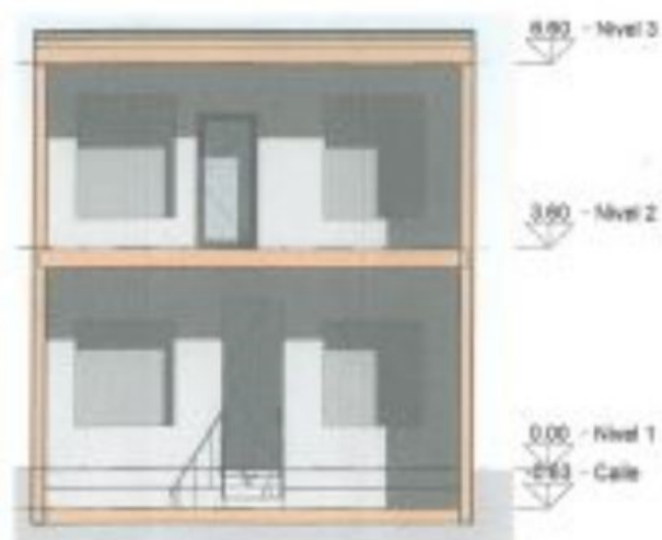
1 Sección 1 Alto: 1:100
