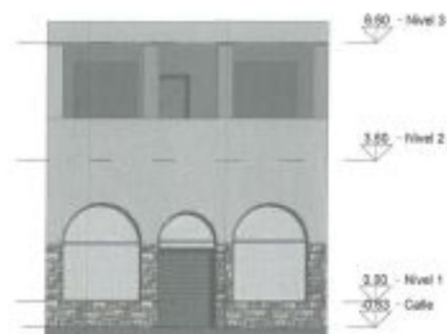
4 Sección Alto: 1:100
