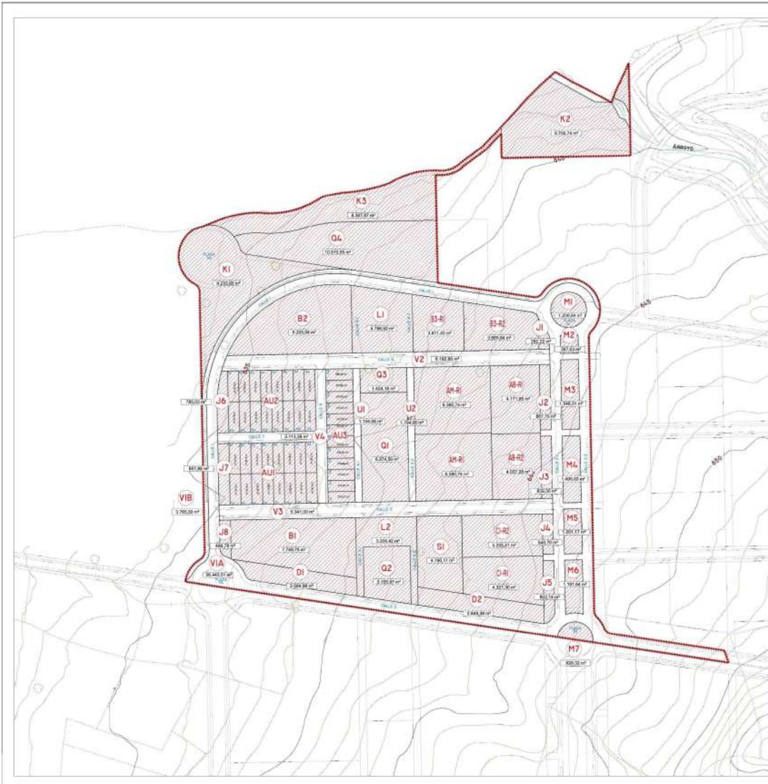
DETALLE DE PLANTA ESCALA: 1:1.000
