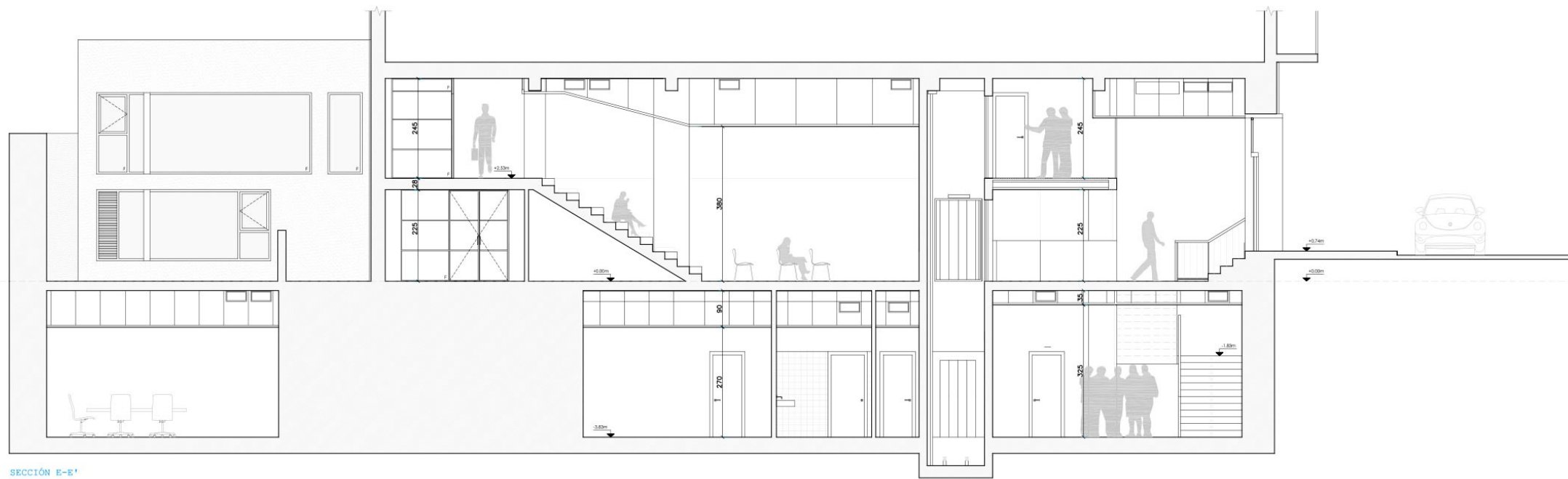
SECCIÓN E-E'
