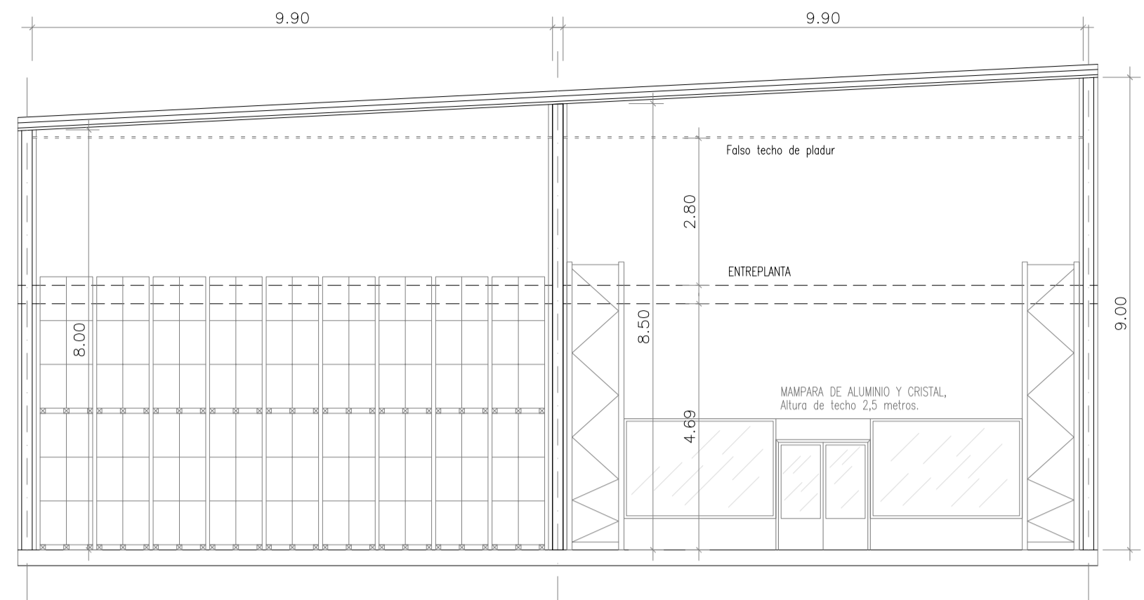
SECCIÓN OP (Estado reformado) ESCALA 1:100
