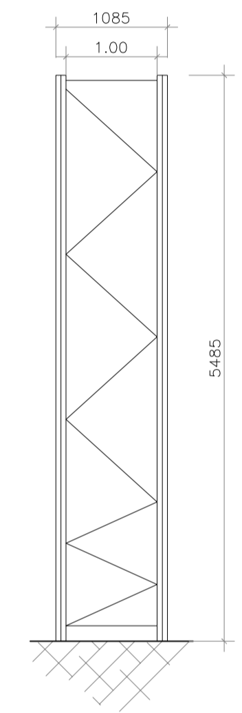
ALZADO LATERAL ESCALA 1:50
