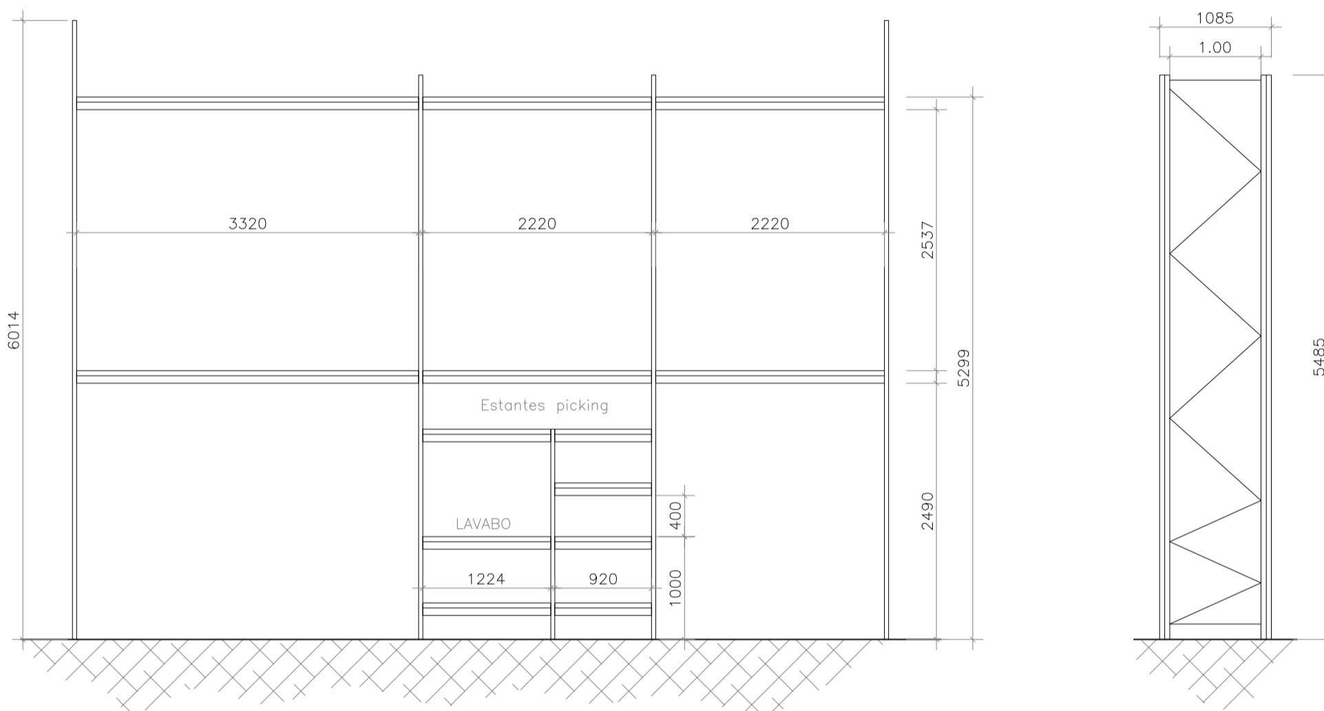
ALZADO FRONTAL ESCALA 1:50
