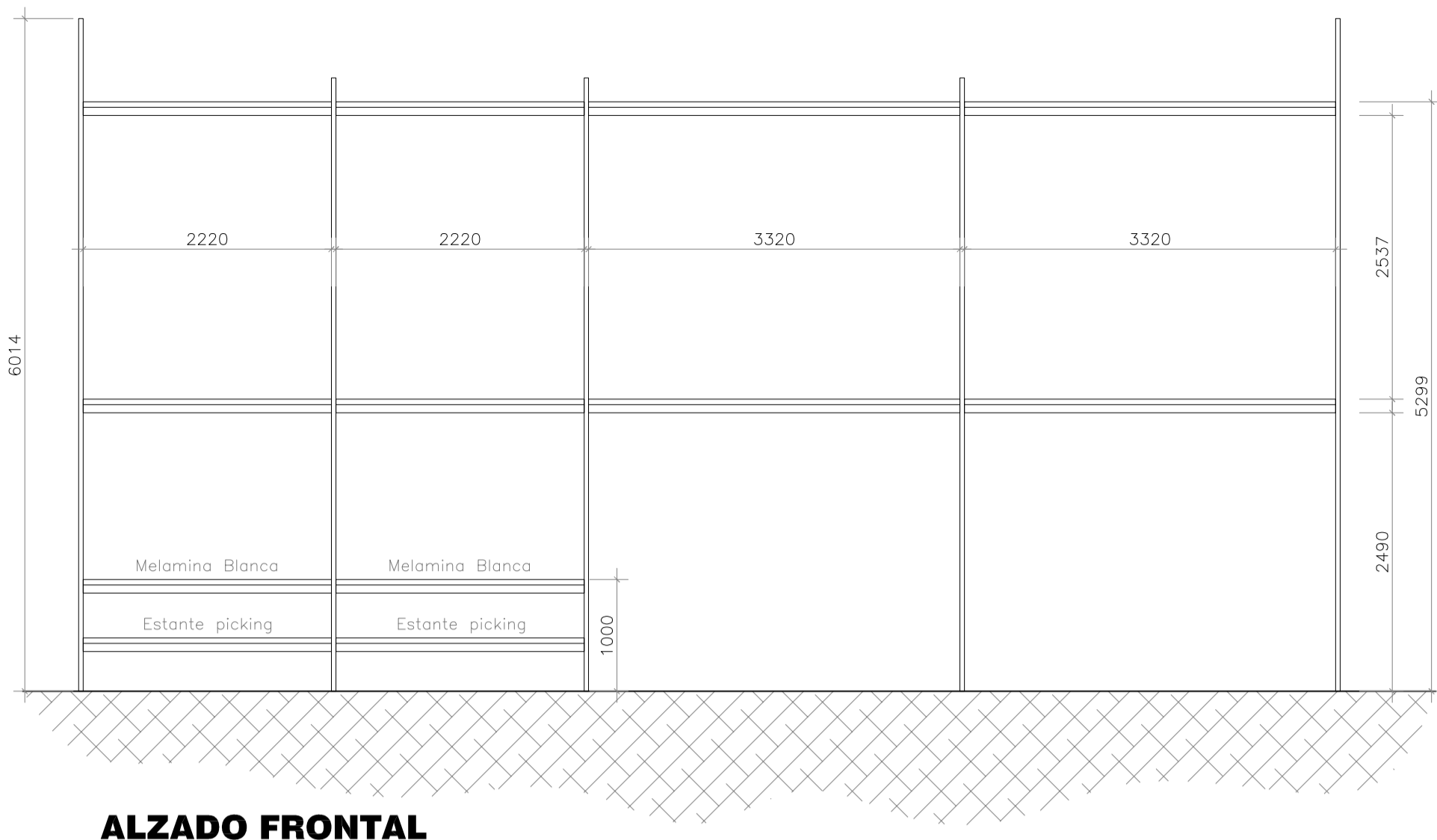
ALZADO FRONTAL ESCALA 1:50
