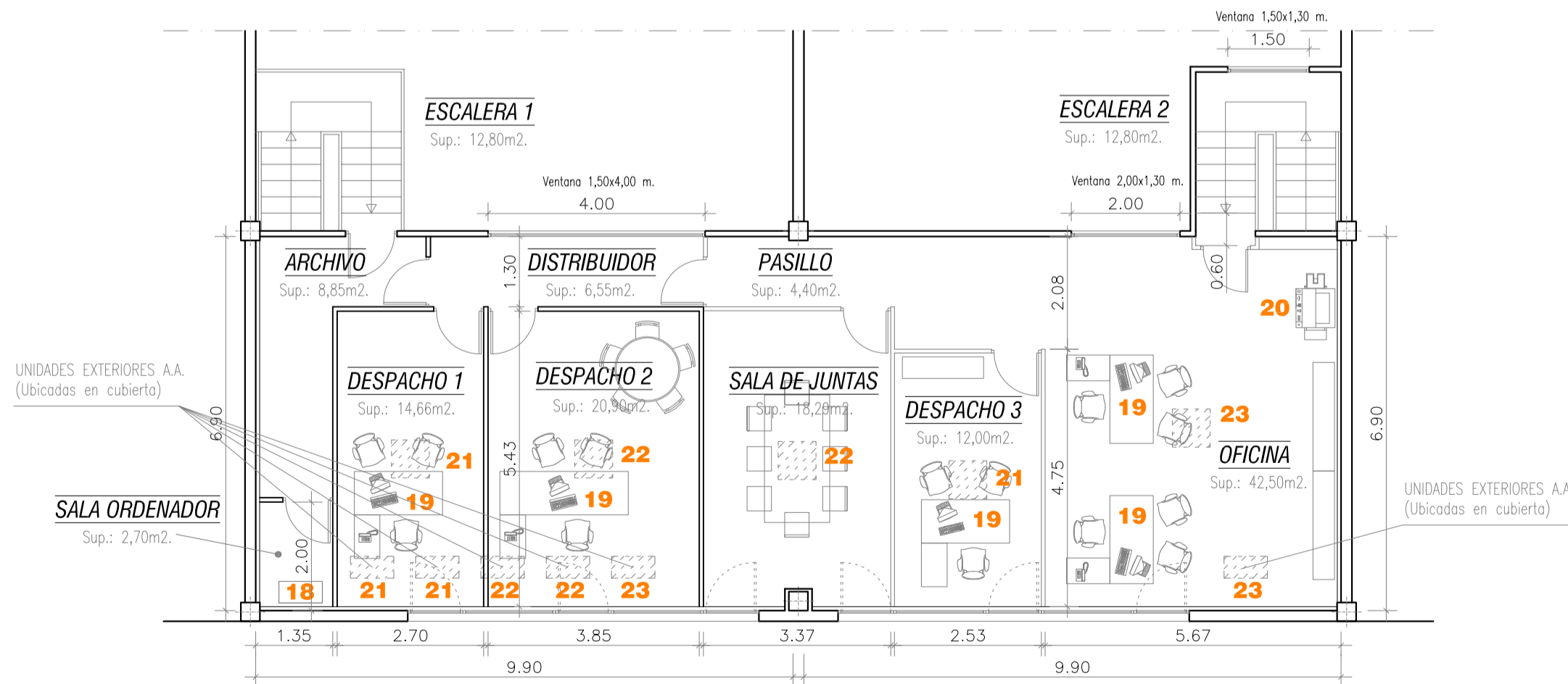
ENTREPLANTA (Cotas, Usos, Mobiliario y Maquinaria) ESCALA 1:100
