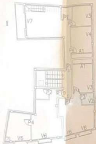
PLANTA PRIMERA
