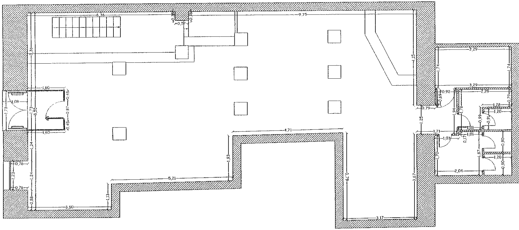
PLANTA BAJA 144,80 m 2 e 1:100
